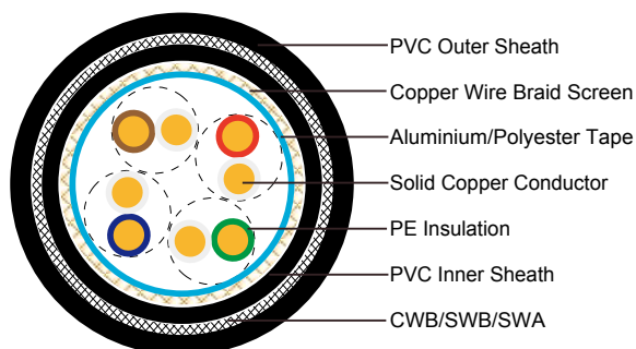
SF/UTP CAT5E
