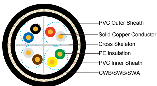
U/UTP CAT6
