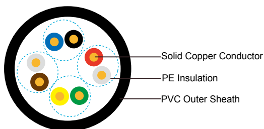
U/UTP CAT5E
