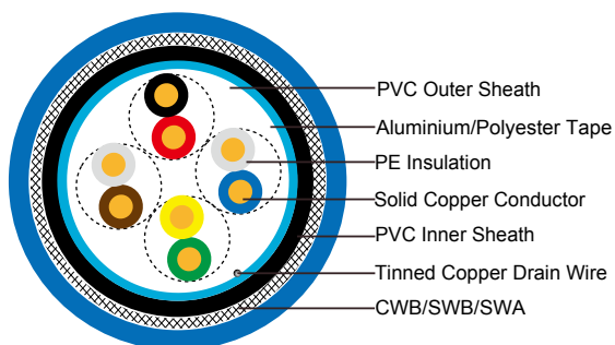
F/UTP CAT5E
