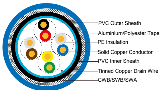
F/UTP CAT6
