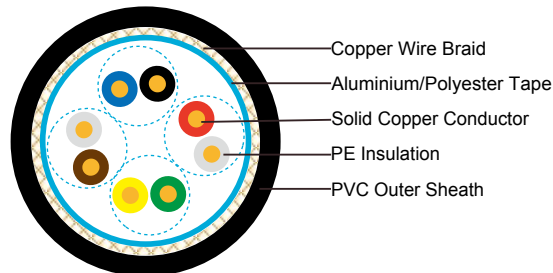
SF/UTP CAT5E
